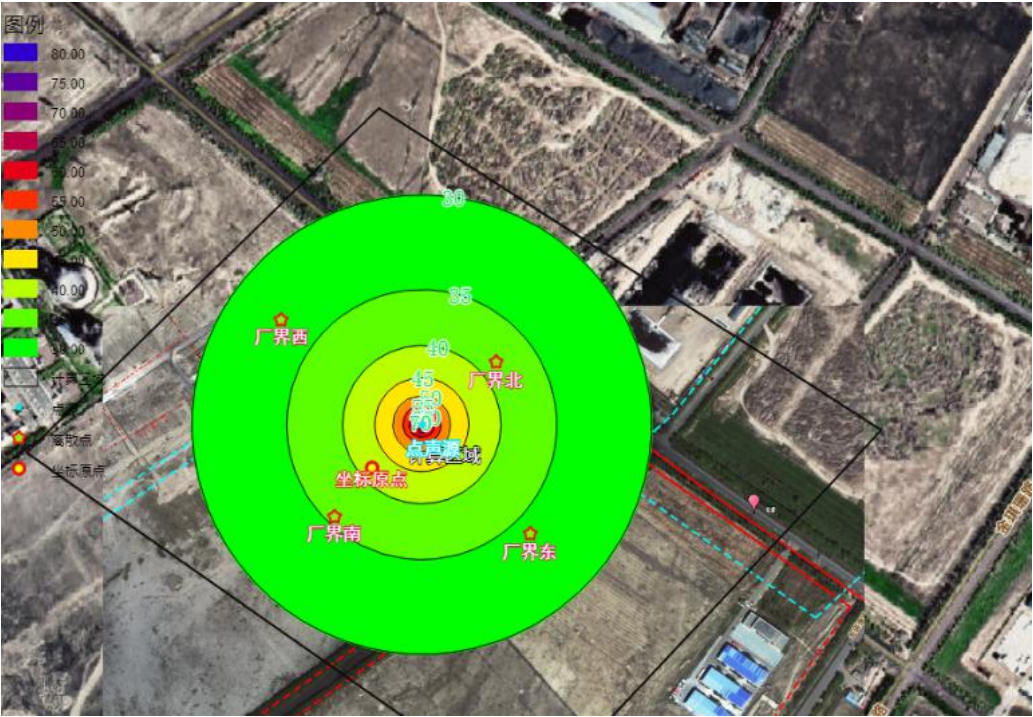
图 4-1 噪声计算等值线图
