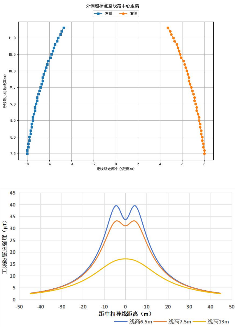
图 3-3 双回路线路正相序工频磁感应强度预测分布曲线（2F2Wb-ZT1 塔型）
