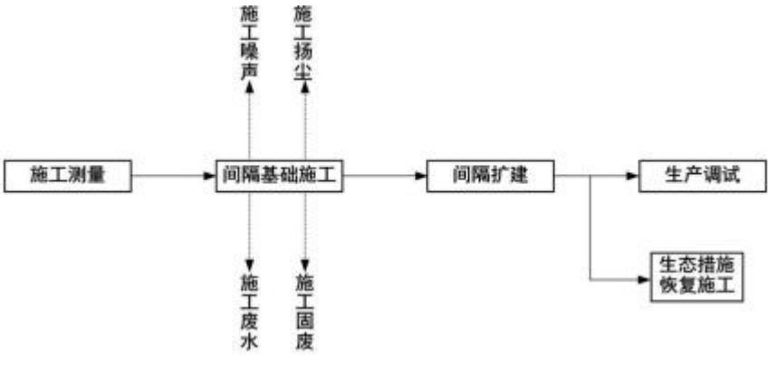
图 2-4 间隔扩建施工工艺流程图
