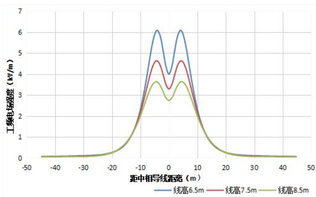
图 3-5 双回路线路逆相序工频电场强度预测分布曲线（2F2Wb-ZT1 塔型）
