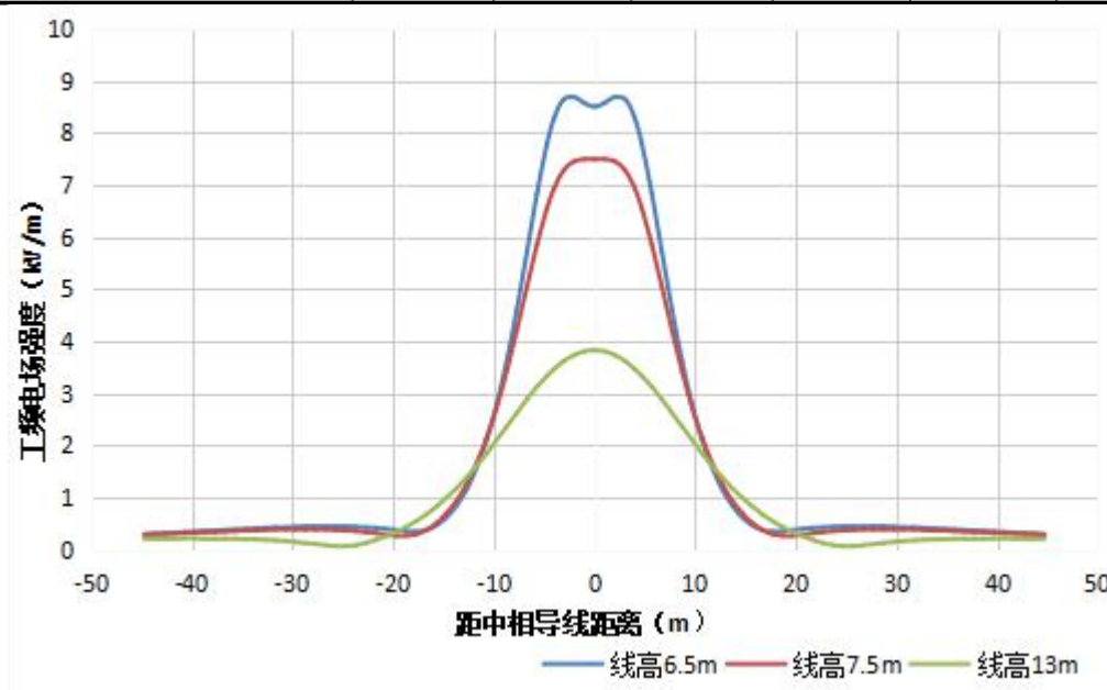
图 3-2 双回路线路正相序工频电场强度预测分布曲线（2F2Wb-ZT1 塔型）
