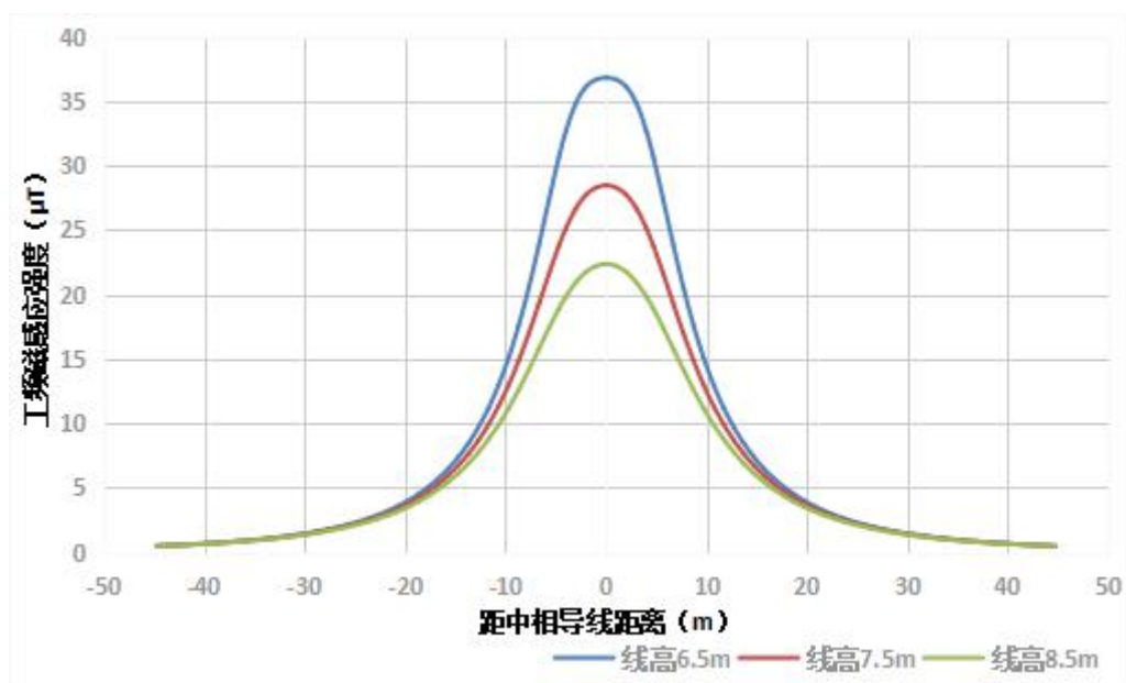
图 3-6 双回路线路逆相序工频磁感应强度预测分布曲线（2F2Wb-ZT1 塔型）
