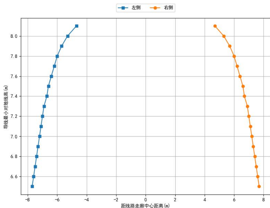
图 3-7 双回路线路逆相序电场强度 4kV/m 等值线预测图
