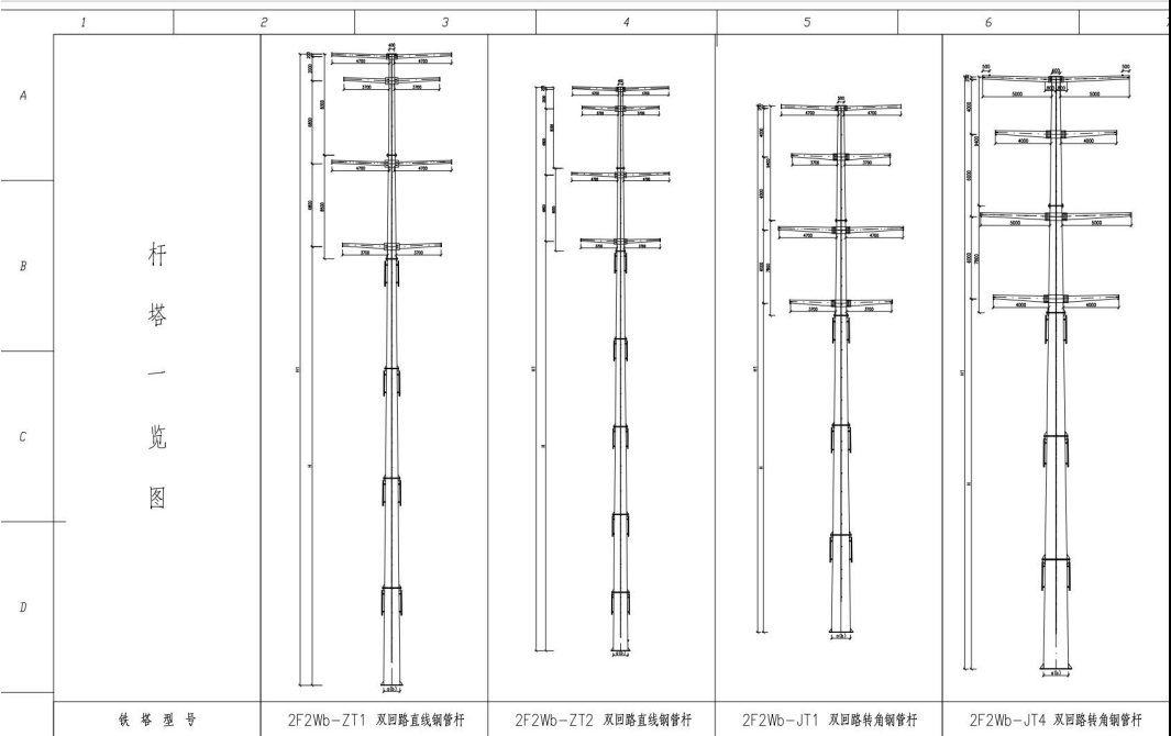
图 2-1 项目塔杆类型一览表
