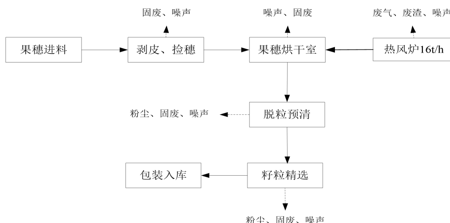
框图 2 项目生产工艺流程及产污节点图
