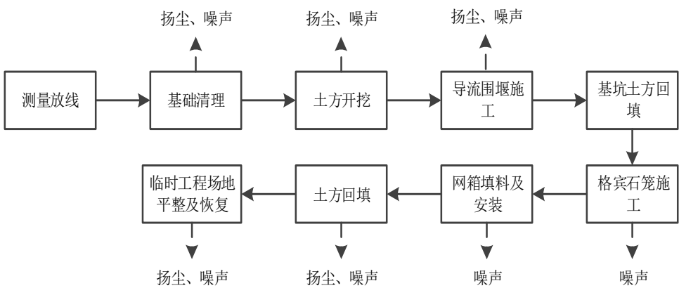
图 2 护岸施工工艺流程图
